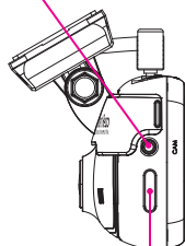
駐車監視スイッチ 1回押す:強制保存 長押 (5秒):駐車監視 ON/OFF切替
